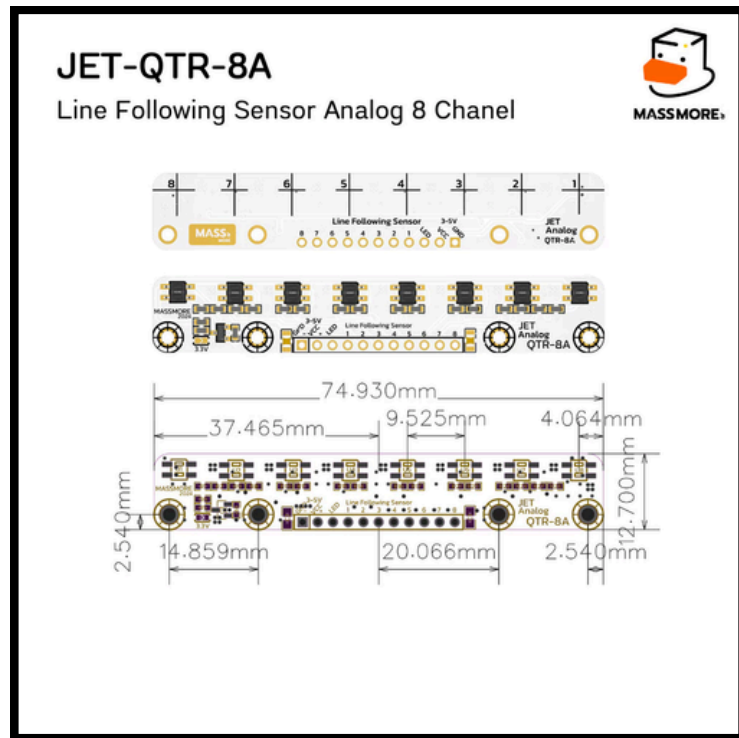
QTR 8A Sensor
